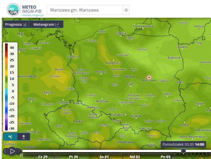
Prognozowana wartość temperatury powietrza na wysokości 2 m nad powierzchnią ziemi w poniedziałek 3 maja 2021 r. o godz. 14:00 wg modelu GFS. | https://meteo.imgw.pl/
