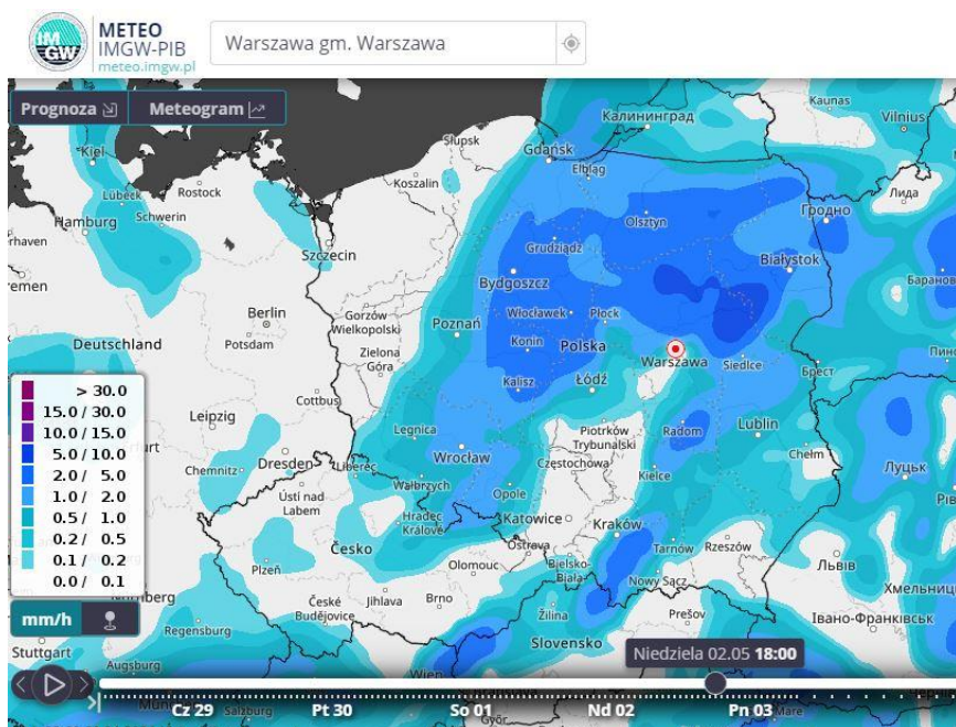
Prognoza opadów deszczu w niedzielę 2 maja 2021 r. o godz. 18:00 wg modelu GFS. | https://meteo.imgw.pl/
