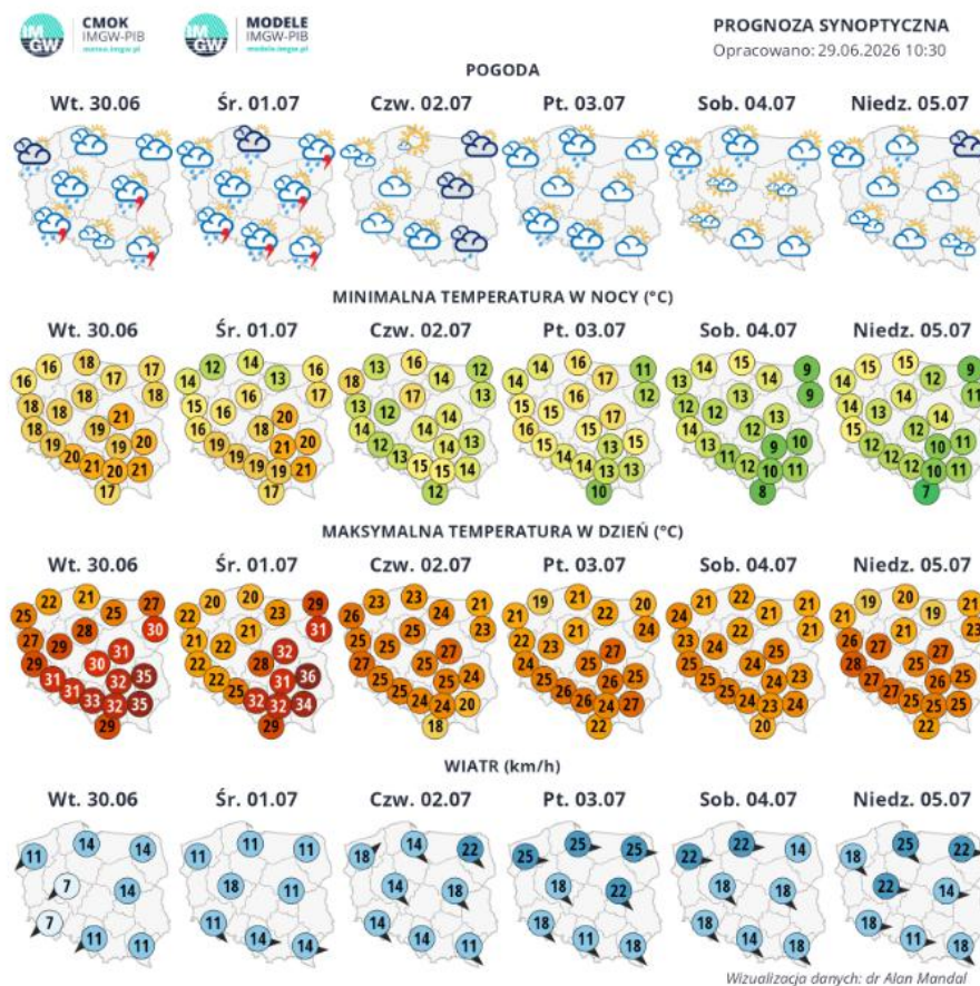
Rys. 1. IMGW_0629 Prognoza synoptyczna na kolejny tydzień 29.06 - 05.07.2026
