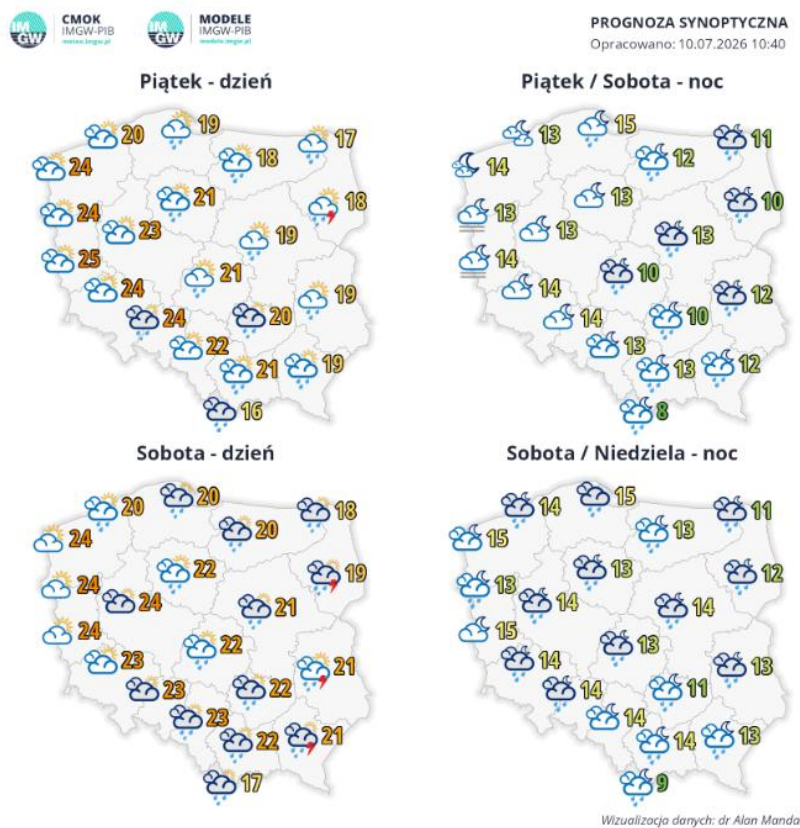
Rys.1 Synoptyczna prognoza pogody na weekend 10-12.07.2026
