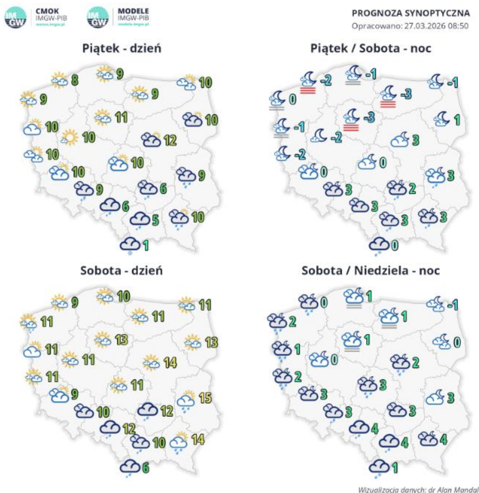
Rys.1. Synoptyczna prognoza pogody na weekend 27-29.03.2026
