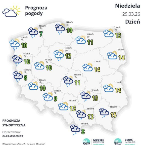
Rys.2. Synoptyczna prognoza pogody na weekend 27-29.03.2026
