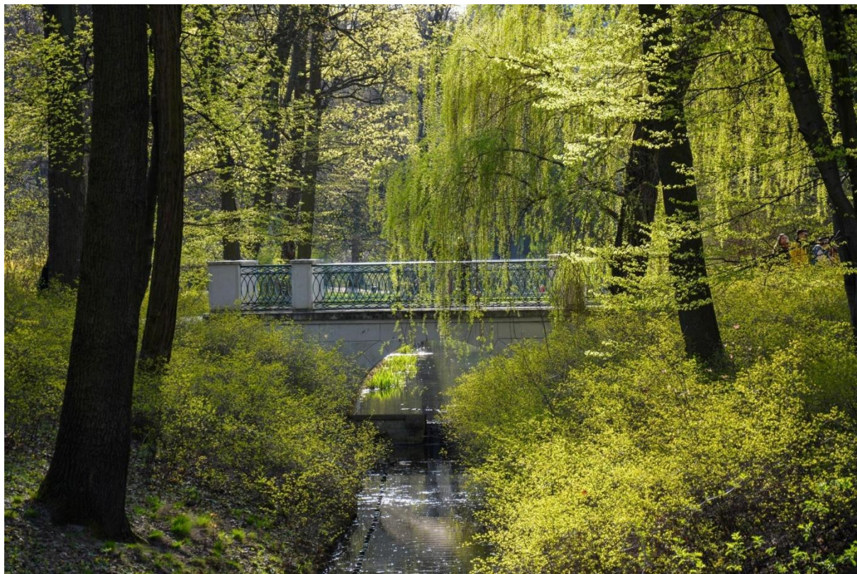
Rys.1 Synoptyczna prognoza pogody na tydzień 13-19.04.2026, fot. Sandra Sowińska-Pazio
