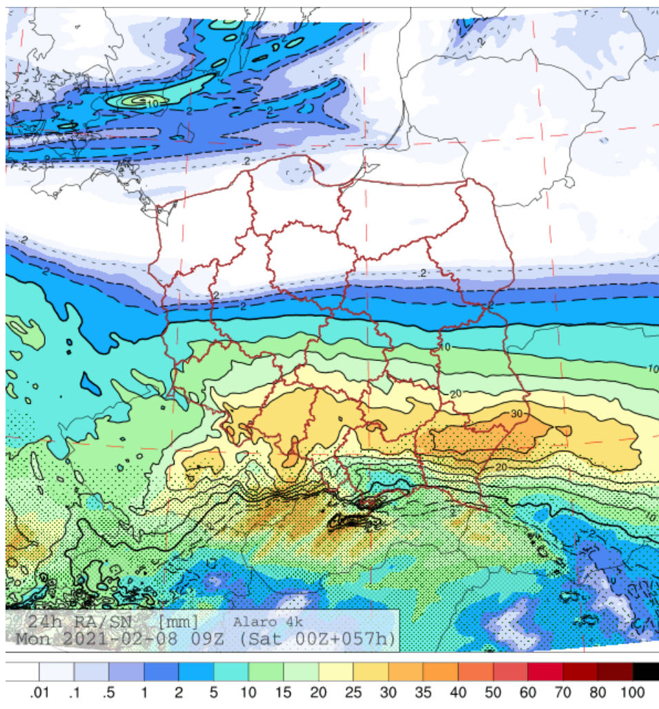
Ryc. 1. Prognozowana wysokość opadów za dobę w poniedziałek 08.02.2021 o godzinie 09:00 UTC (model ALARO).
