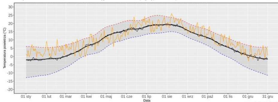
WARSZAWA-OKĘCIE – zmienność średniej dobowej temperatury powietrza (TSRD) w 2020 roku na tle charakterystyk wieloletnich 1981-2010 średnia dobową temperaturę powietrza w 2020 roku (linia pomarańczowa), średnia wieloletnia (linia czarna), kwantyle: 95% (linia czerwona) oraz 5% (linia niebieska) – wygładzone lokalnie ważoną regresją wielomianową
