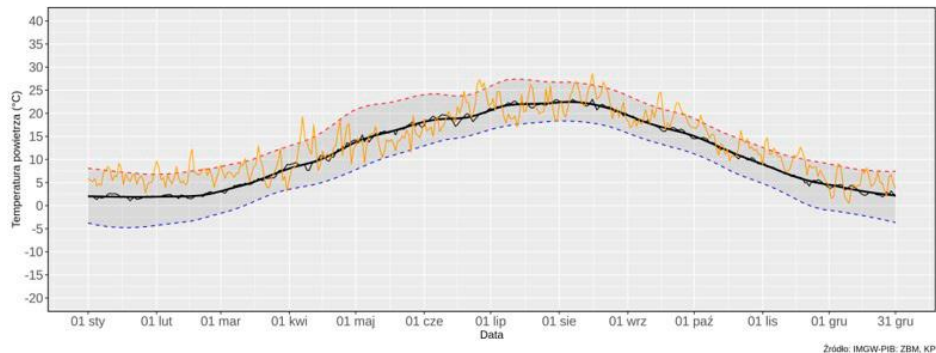
WARSZAWA-OKĘCIE - zmienność maksymalnej dobowej temperatury powietrza (TMAX) w 2020 roku na tle charakterystyk wieloletnich 1981-2010 maksymalna dobową temperaturę powietrza w 2020 roku (linia pomarańczowa), średnia wieloletnia (linia czarna), kwantyle: 95% (linia czerwona) oraz 5% (linia niebieska) – wygładzone lokalnie ważoną regresją wielomianową
