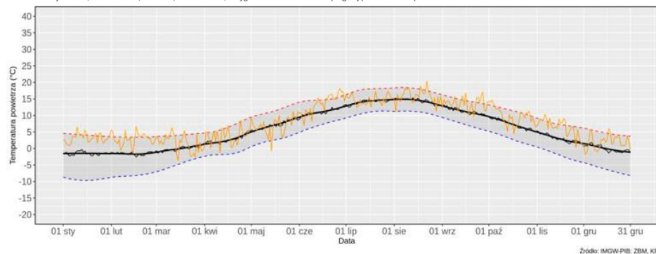
WARSZAWA-OKĘCIE - zmienność minimalnej dobowej temperatury powietrza (TMIN) w 2020 roku na tle charakterystyk wieloletnich 1981-2010 minimalna dobowa temperatura powietrza w 2020 roku (linia pomarańczowa), średnia wieloletnia (linia czarna), kwantyle: 95% (linia czerwona) oraz 5% (linia niebieska) – wygładzone lokalnie ważoną regresją wielomianową
