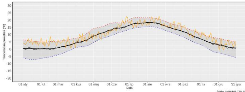
WARSZAWA-OKĘCIE – zmienność średniej dobowej temperatury powietrza (TSRD) w 2020 roku na tle charakterystyk wieloletnich 1981-2010 średnia dobową temperaturę powietrza w 2020 roku (linia pomarańczowa), średnia wieloletnia (linia czarna), kwantyle: 95% (linia czerwona) oraz 5% (linia niebieska) – wygładzone lokalnie ważoną regresją wielomianową
