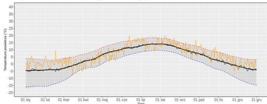
KROSNO - zmienność minimalnej dobowej temperatury powietrza (TMIN) w 2020 roku na tle charakterystyk wieloletnich 1981-2010 minimalna dobowa temperatura powietrza w 2020 roku (linia pomarańczowa), średnia wieloletnia (linia czarna), kwantyle: 95% (linia czerwona) oraz 5% (linia niebieska) – wygładzone lokalnie ważoną regresją wielomianową
