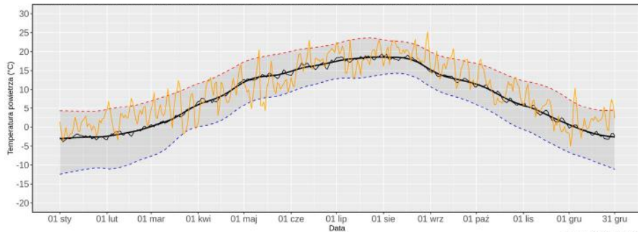
KROSNO – zmienność średniej dobowej temperatury powietrza (TSRD) w 2020 roku na tle charakterystyk wieloletnich 1981-2010 średnia dobową temperaturę powietrza w 2020 roku (linia pomarańczowa), średnia wieloletnia (linia czarna), kwantyle: 95% (linia czerwona) oraz 5% (linia niebieska) – wygładzone lokalnie ważoną regresją wielomianową
