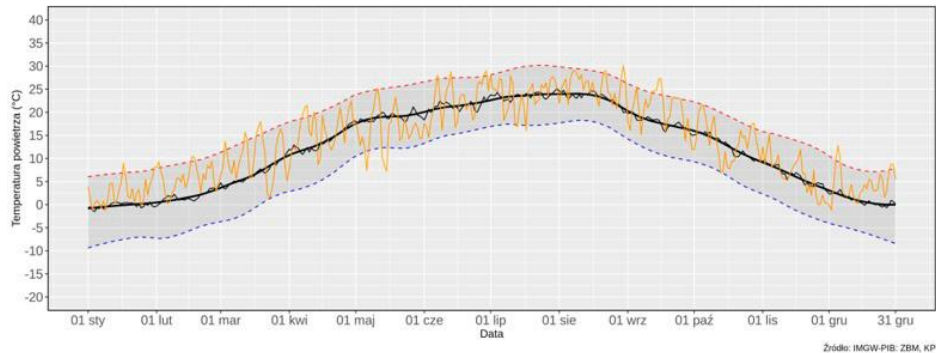
KROSNO - zmienność maksymalnej dobowej temperatury powietrza (TMAX) w 2020 roku na tle charakterystyk wieloletnich 1981-2010 maksymalna dobową temperaturę powietrza w 2020 roku (linia pomarańczowa), średnia wieloletnia (linia czarna), kwantyle: 95% (linia czerwona) oraz 5% (linia niebieska) – wygładzone lokalnie ważoną regresją wielomianową
