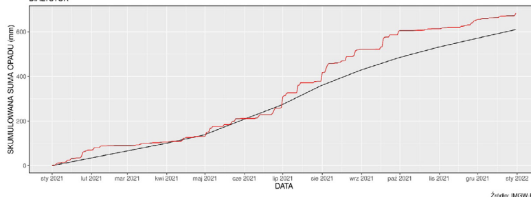
Skumulowane dobowe sumy opadu w roku 2021 - linia czerwona na tle kumulowanych norm wieloletnich 1991-2020 - linia czarna CHOJNICE
