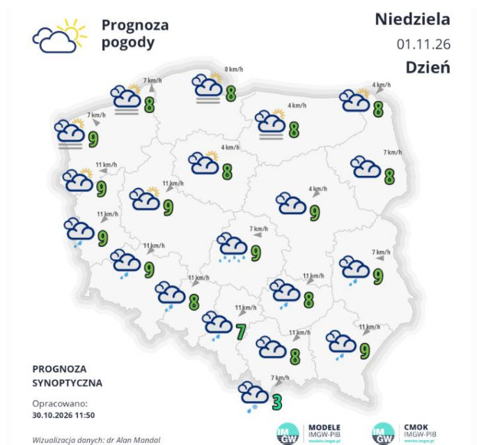
Ryc.2. IMGW_1030_synoptyczna prognoza pogody na weekend 30.10-02.11.10.2026
