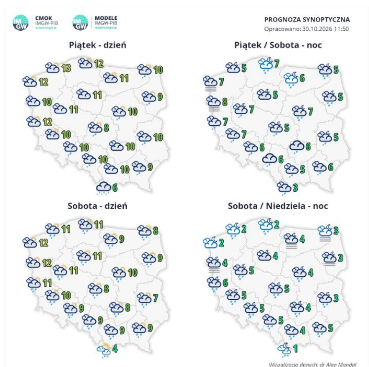
Ryc.1. IMGW_1030_synoptyczna prognoza pogody na weekend 30.10-02.11.10.2026
